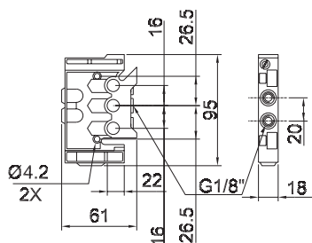
Simple piloto
