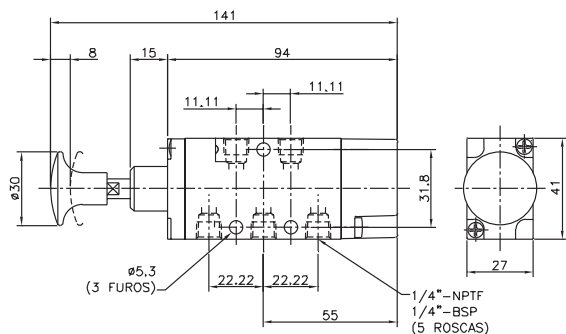
Válvula botão/mola
