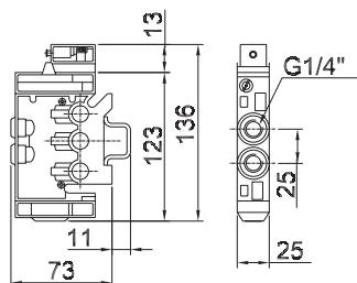
Simple piloto
