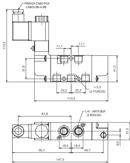
Válvula Solenoide/piloto
