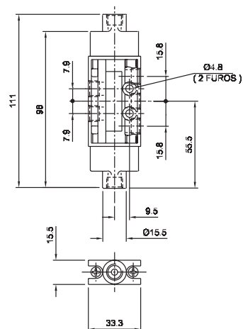
Válvula rolete/mola - 5/2 vias
