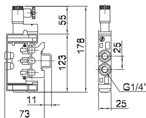
Simple solenóide
