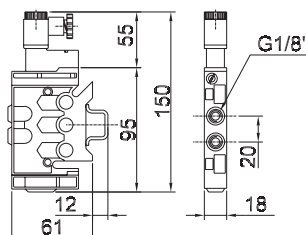
Simple solenóide
