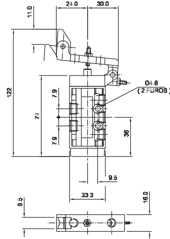
Válvula pino/mola - 5/2 vias
