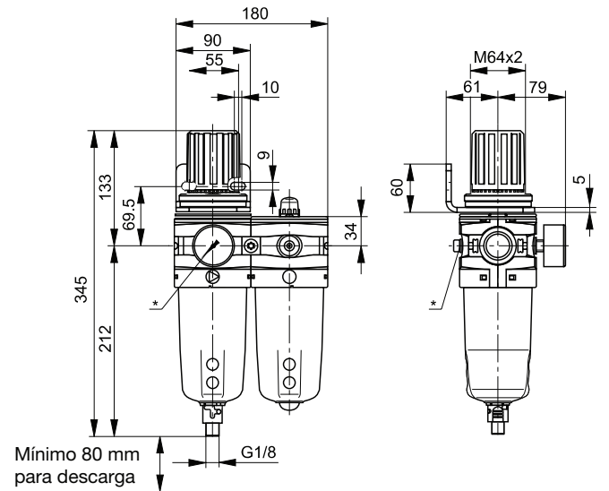
Conjunto montado FR + L
