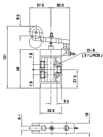
Válvula rolete/mola - 3/2 vias
