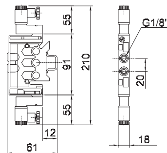
Duplo solenóide
