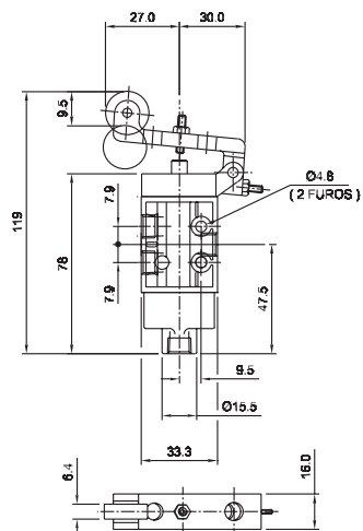
Válvula rolete/piloto - 3/2 vias
